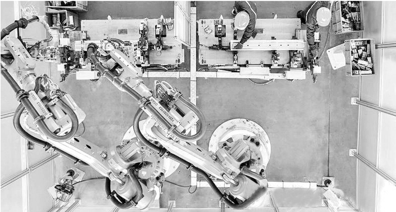
8月17日,位于浙江省湖州市长兴经济技术开发区的一家汽车部件有限公司数字车间内全自动机器人正在高速运转,赶制一家汽车厂商的白车身前机舱订单产品。该公司通过数字化改革打造智慧工厂,投资1亿多元引进近百台(套)ABB点焊自动化工作站、安川弧焊机机器人,全链融合智能传感器、分析技术与人工智能,实现全线数字化智能化生产,助力提质增效,为长三角汽车及零部件产业强链、补链注入强劲动能。
